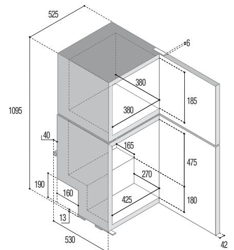
Dimensioni versione standard (senza profilo di fissaggio) Standard version dimensions (no mounting flange)
